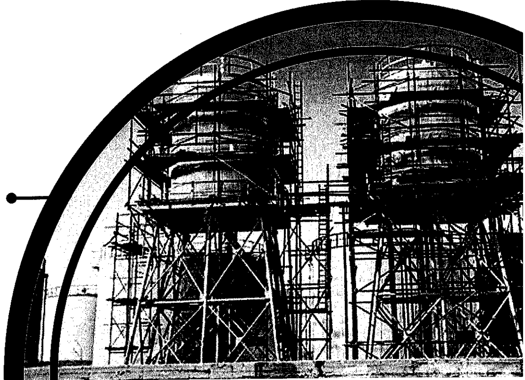
اعمال السقالات لمشروع الصيانة الشاملة لمصهارج سعات مختلفة بحقول الصحراء الغربية لصالح الشركة العامة للبترول
